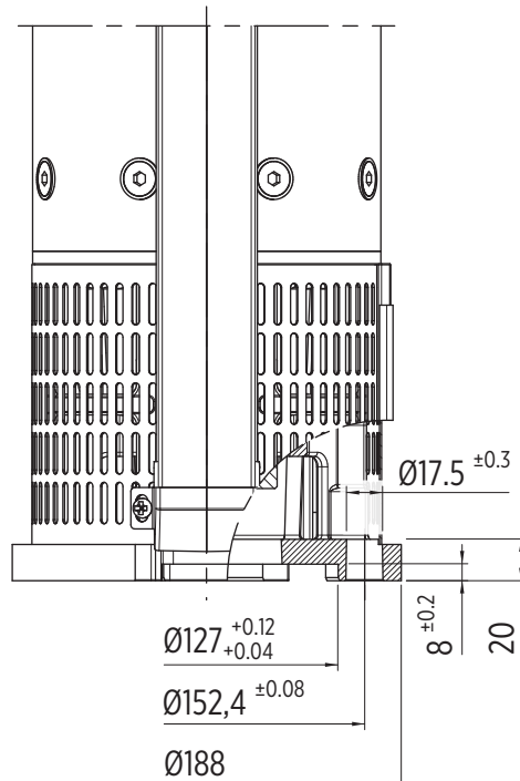
6" MOTORADAPTER FÜR I, N UND R VERSION
