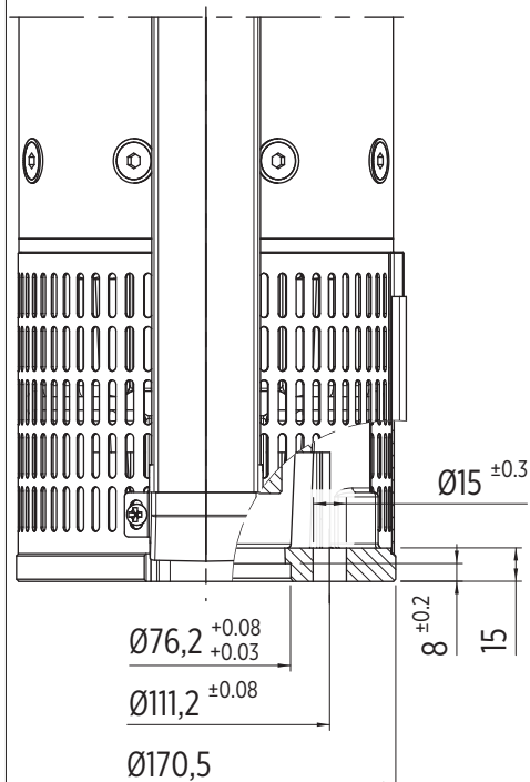
4" MOTORADAPTER FÜR I UND N VERSION
