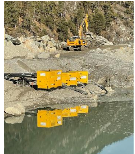
Dieselmotorpumpen im Einsatz S150D, S200D
